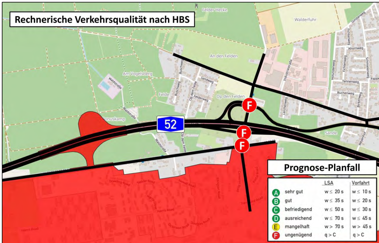
Abbildung 23: Rechnerische Verkehrsqualität im Prognose-Planfall (Kartengrundlage: [1])
