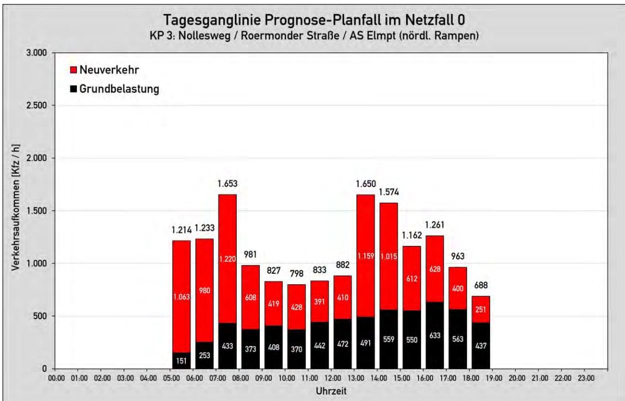
Abbildung 20: Tagesganglinie am Knotenpunkt Nollsweg / Roermonder Straße / AS Elmpt (nördl. Rampen) (KP 3) im Prognose-Planfall
