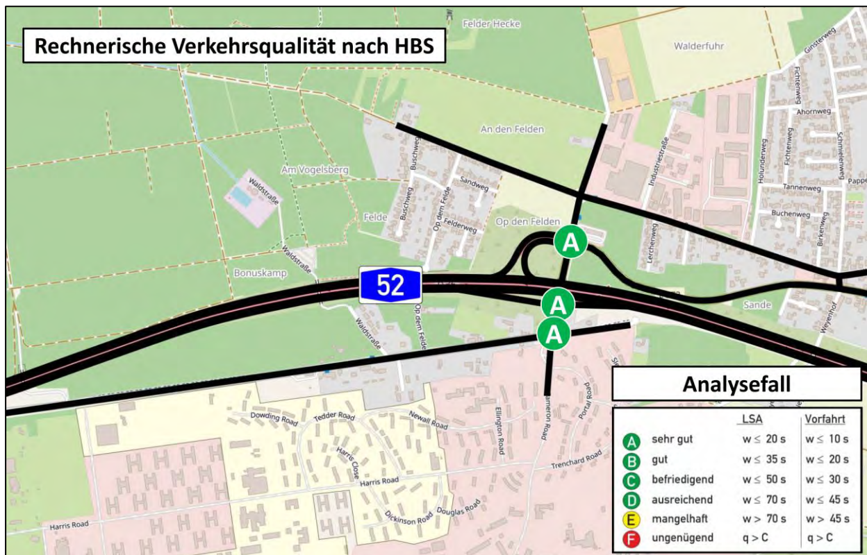
Abbildung 21: Rechnerische Verkehrsqualität im Analysefall (Kartengrundlage: [1])
