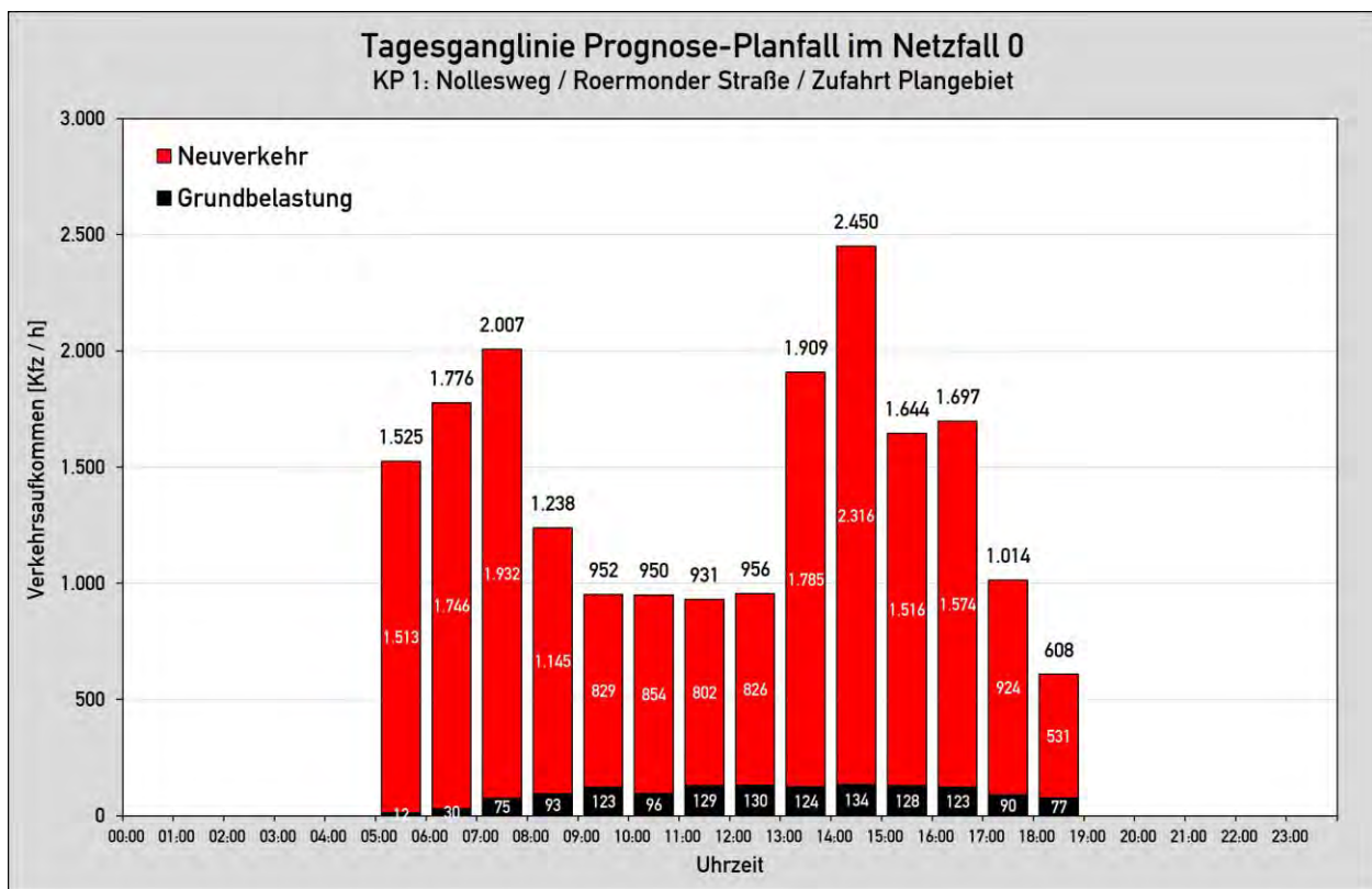
Abbildung 18: Tagesganglinie am Knotenpunkt Nollesweg / Roermonder Straße / Zufahrt Plangebiet (KP 1) im Prognose-Planfall
