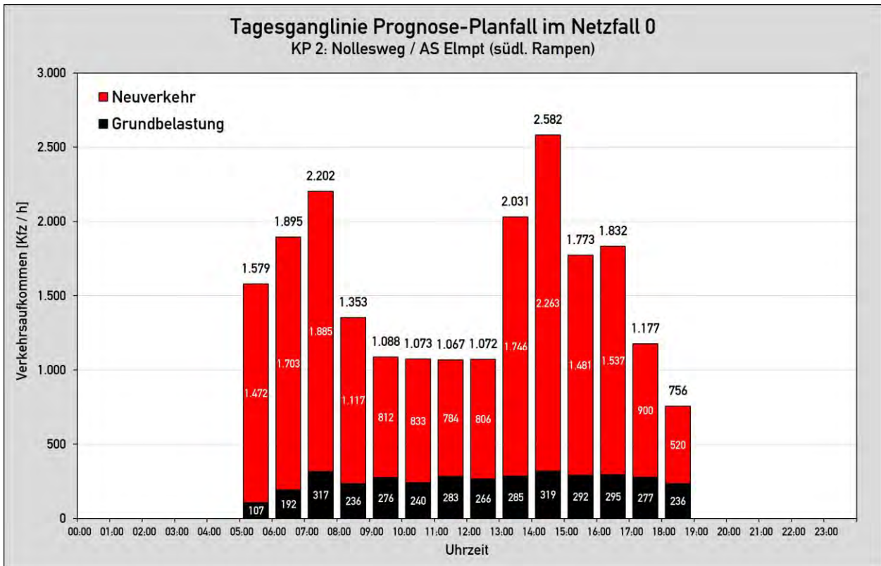
Abbildung 19: Tagesganglinie am Knotenpunkt Nollsweg / AS Elmpt (südl. Rampen) (KP 2) im Prognose-Planfall
