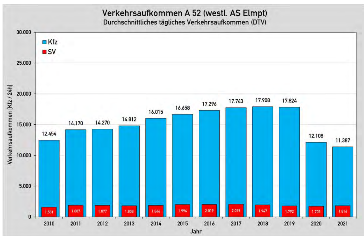
Abbildung 7: Verkehrsentwicklung auf der A 52
