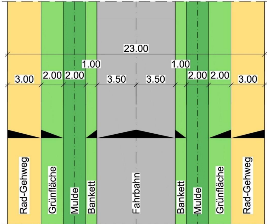
Lageplanausschnitt Bereich RQ1 (Schemadarstellung)
