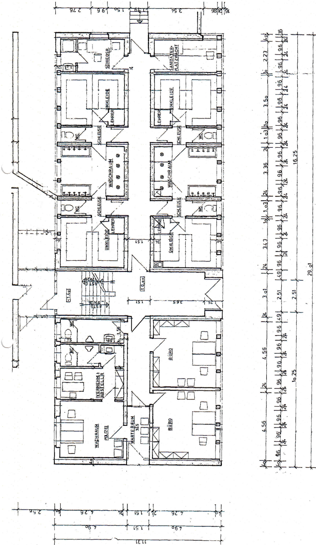
Grundriss ERDGESCHOSS Am Kamp 23
